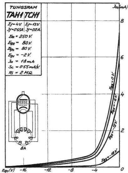
Kennlinien der TAH 1
